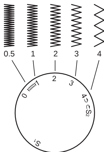
Stichlängenknopf (5)
